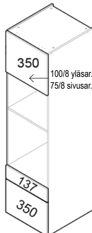
MIKROALTOUUNI + UUNI 2 LTK
