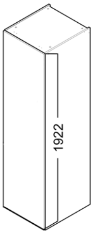
INTEGROITU 1-OVINEN JK/PK • ovi 1920*596 • ei saranaporausta, varmistettava konekohtainen tieto
