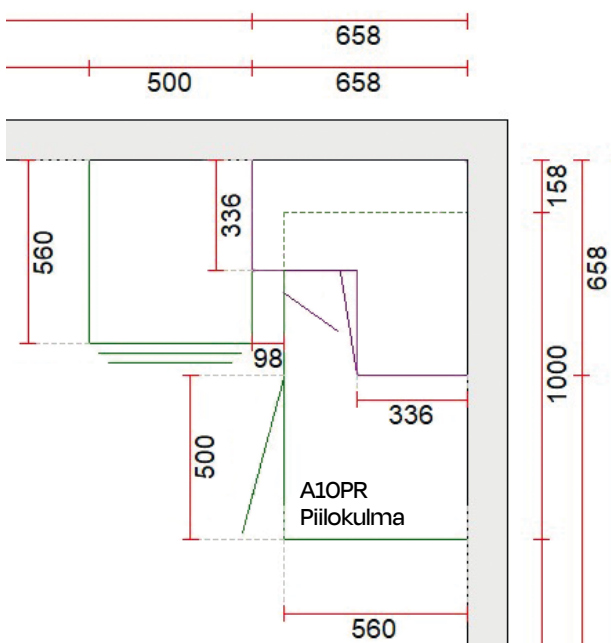
7. Piilokulma mitoitus 1000 mm 496 mm ovella
