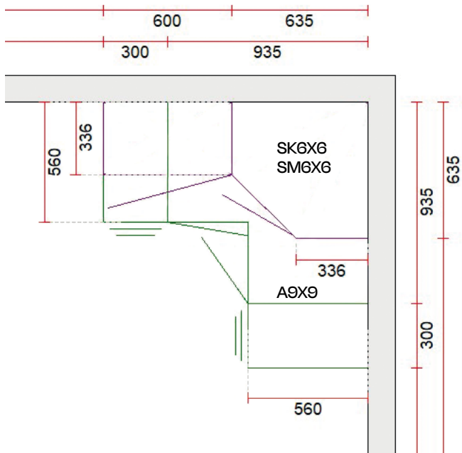
1. Ala- ja yläkulmakaapin mitoitus 935*935 & 635*635 mm
