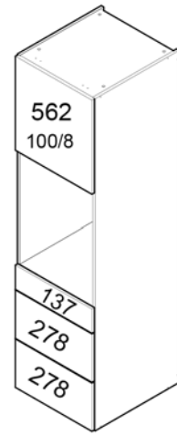
UUNI 3 LAATIKOLLA
