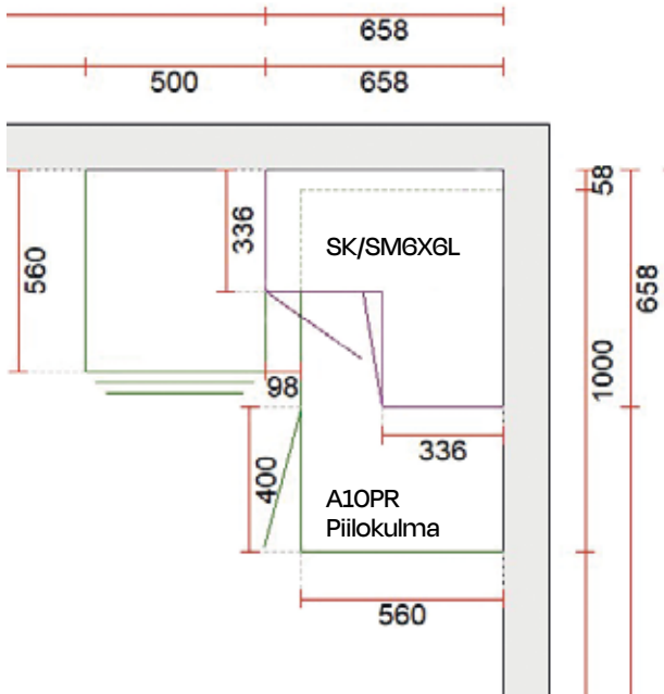
5. Piilokulma mitoitus 1000 mm 396 mm ovella
