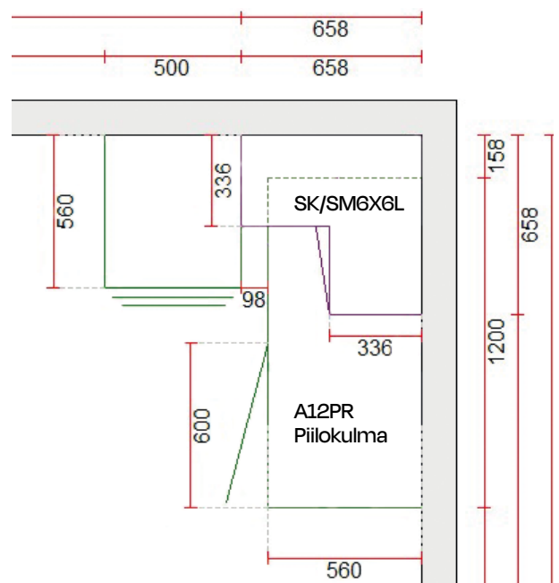
6. Piilokulma mitoitus 1200 mm 596 mm ovella
