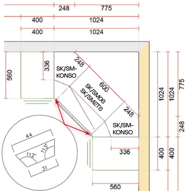
3. Kulmakaapin mitoitus liesikulma 600 mm
