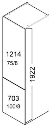
INTEGROITU JK/PK • ovien saranaporaukset varmistettava konekohtaisesti
