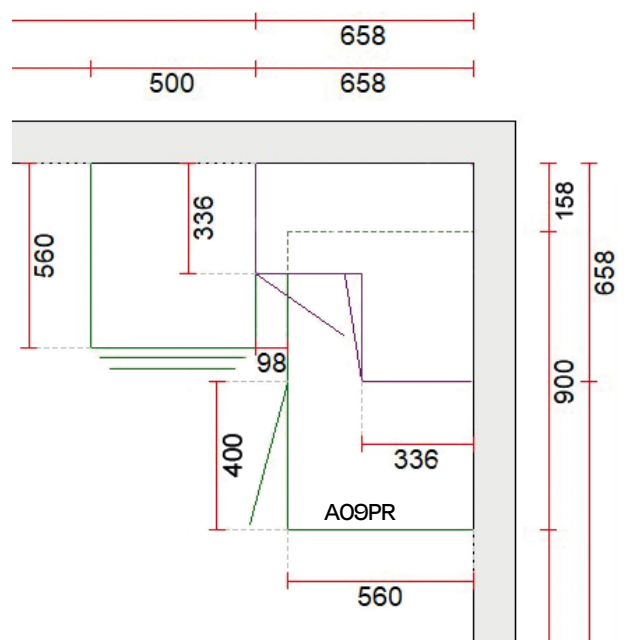
4. Piilokulma mitoitus 900 mm 396mm ovella
