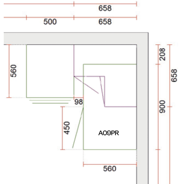
2. Piilokulma 900 mm 446 mm ovella
